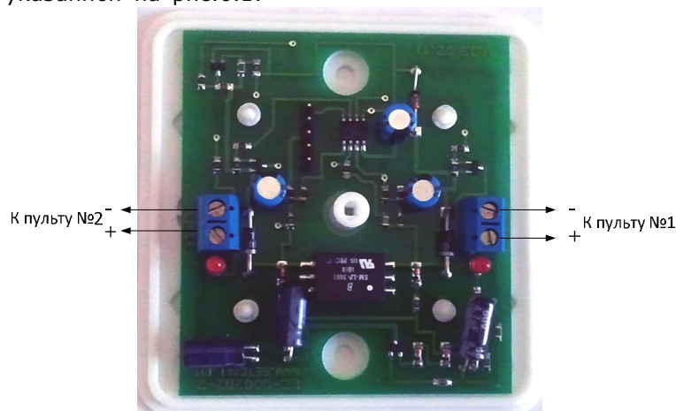
Рисунок 6.1. Внешний вид GC-0002D1 (со снятой крышкой)
