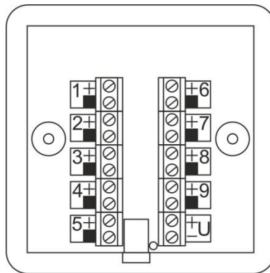
Рисунок 4.2. Внешний вид коммутационной коробки при снятой крышке
