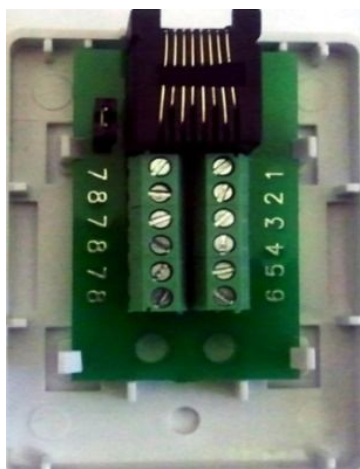
Рисунок 4.1. Внешний вид монтажной коробки GC-0009U1 при снятой крышке
